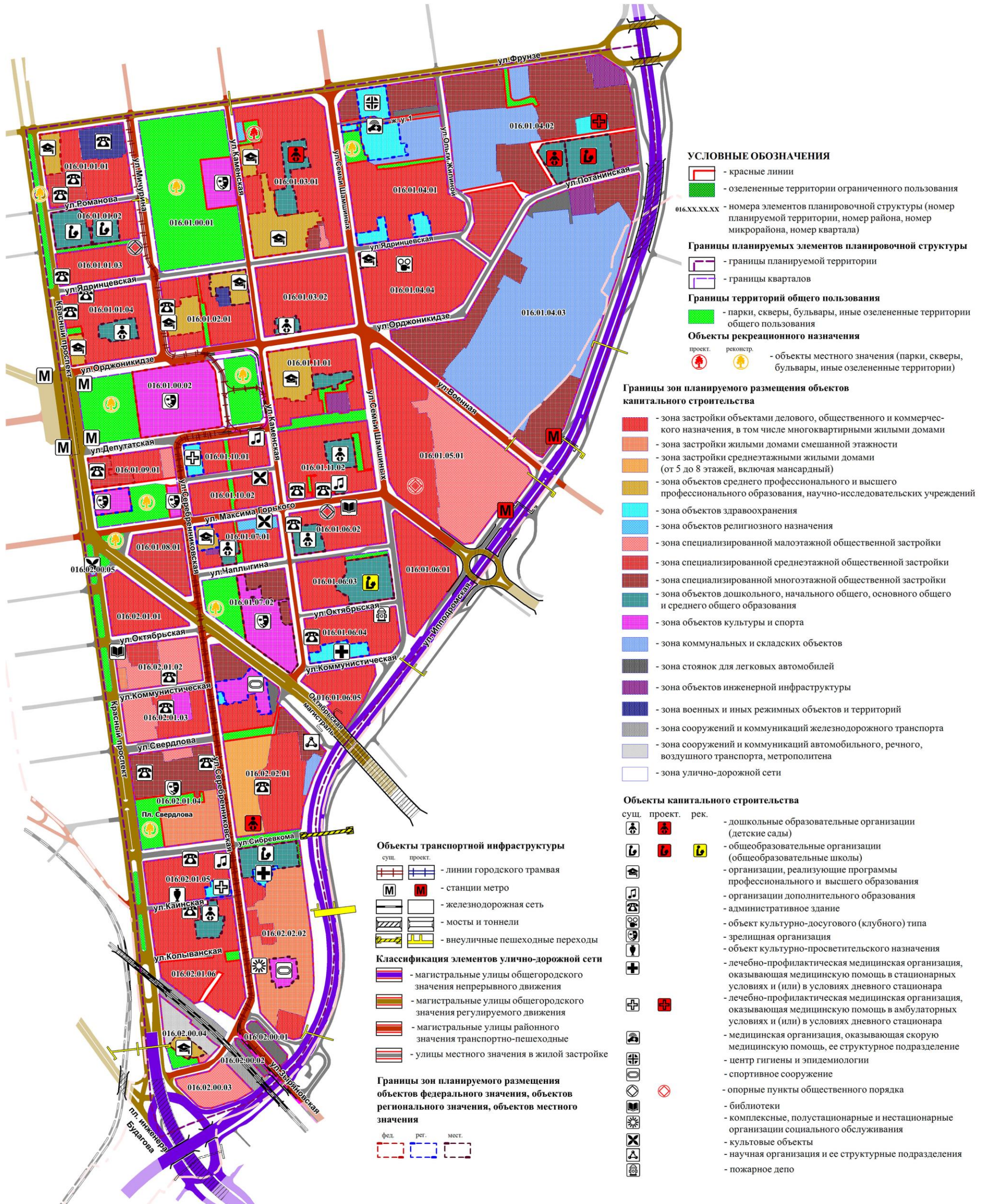
ЧЕРТЕЖ планировки территории
